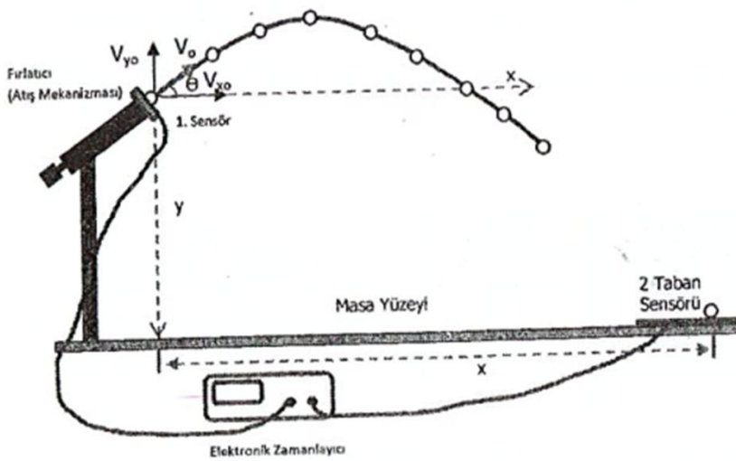
Şekil 4. Elektronik Zamanlayıcı kullanılarak yatay olarak fırlatılan bir cismin ilk hızını belirleyecek deney ...
