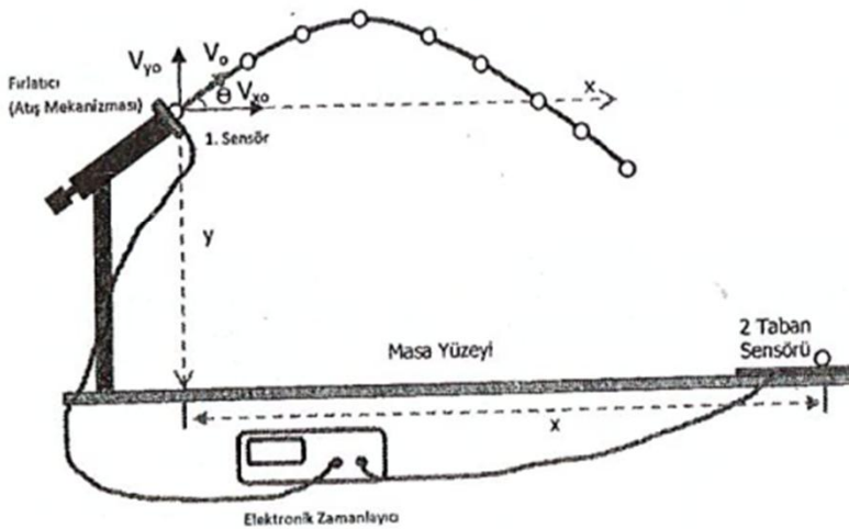
Şekil 4. Elektronik Zamanlayıcı kullanılarak yatay olarak fırlatılan bir cismin ilk hızını belirleyecek deney düzeneği
