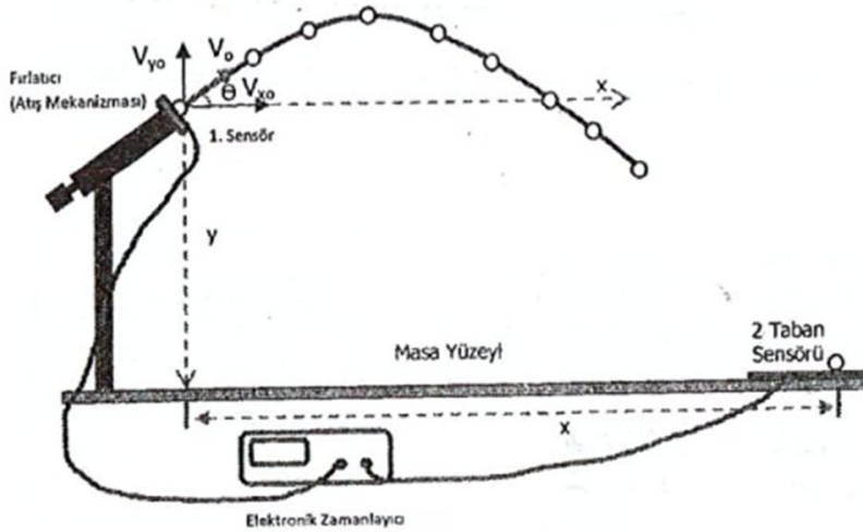
Şekil 4. Elektronik Zamanlayıcı kullanarak yatay olarak fırlatılan bir cismin ilk hızını belirleyecek deney düzeneği
