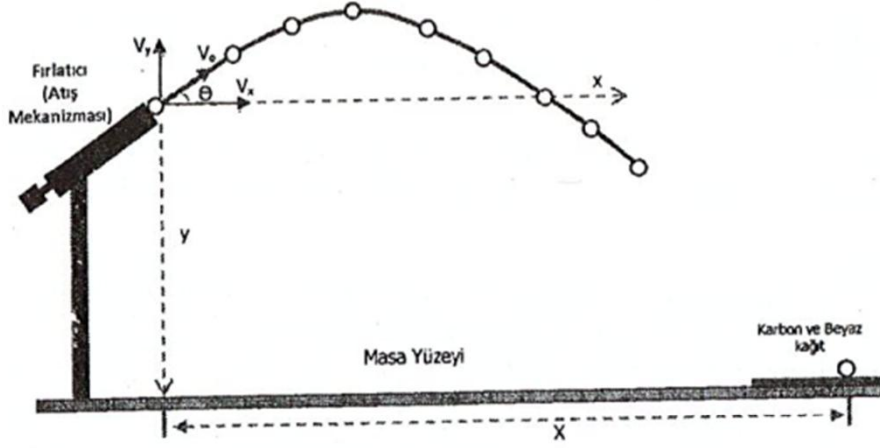
Şekil 3. Yatay eksene göre belirli bir açı ile fırlatılan bilyenin aldığı yatay mesafeyi bulmak için hazırlanan deney düzeneği
