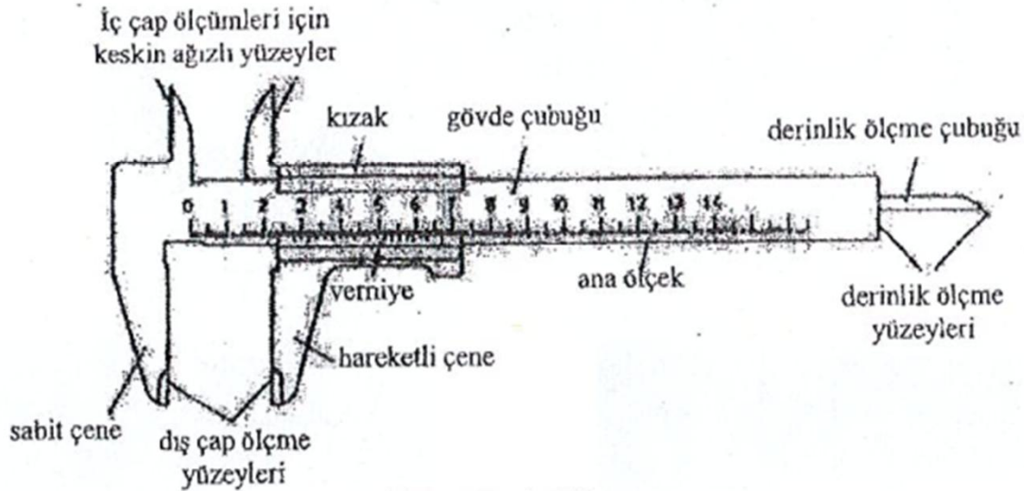
Şekil 1. Verniyeli Kumpas
